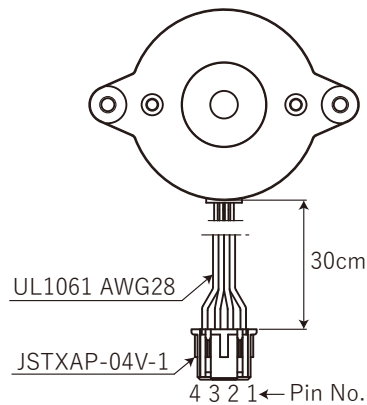
モータ結線図
